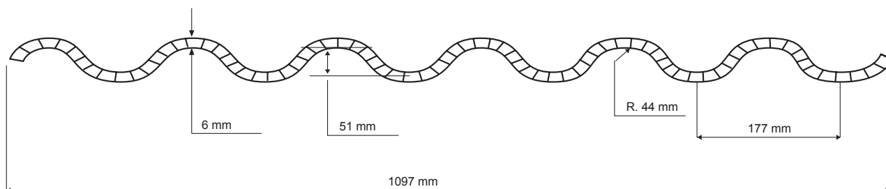
SEZIONE LASTRA: PASSO EUROPEO SEI ONDE E MEZZO
